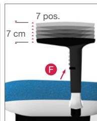
Regulació del braç en altura 7 posicions
